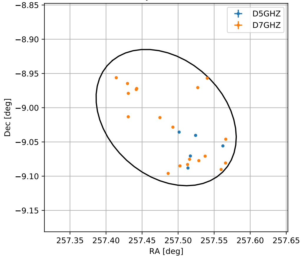
4FGL J1709.9-0900
