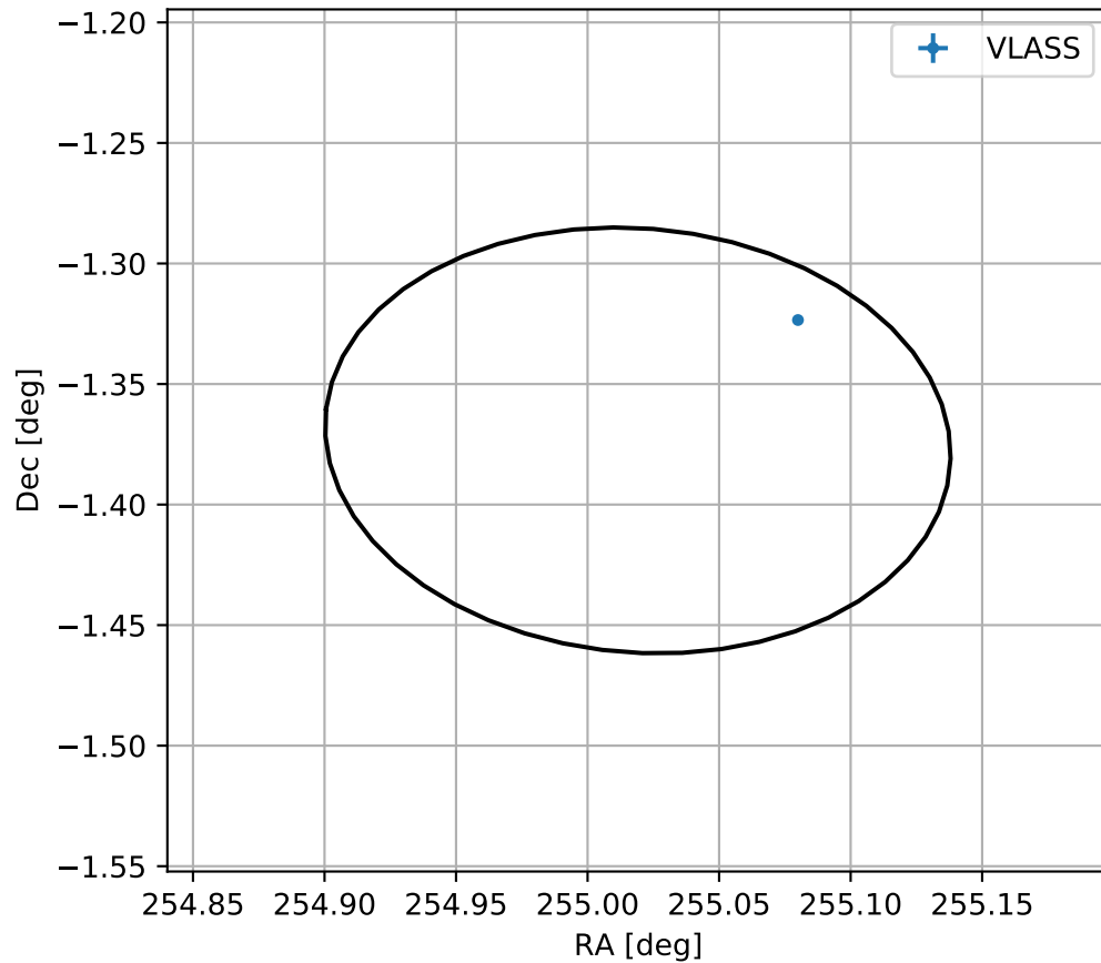
4FGL J1700.0-0122
