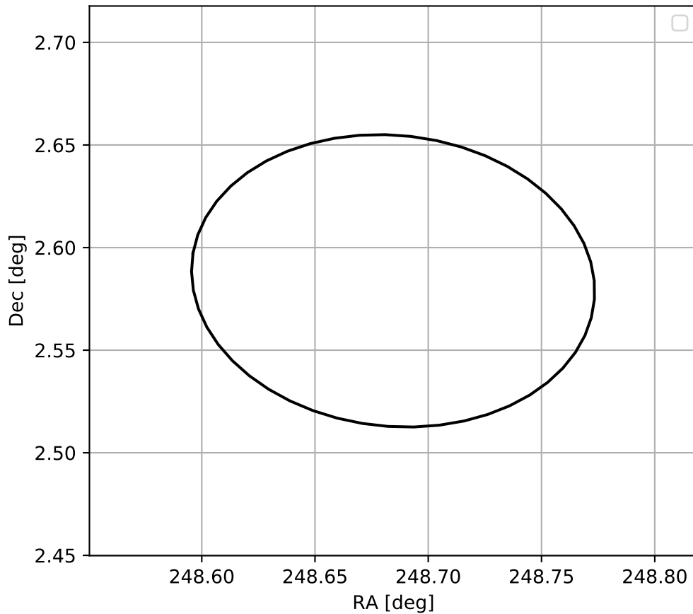
4FGL J1634.7+0235
