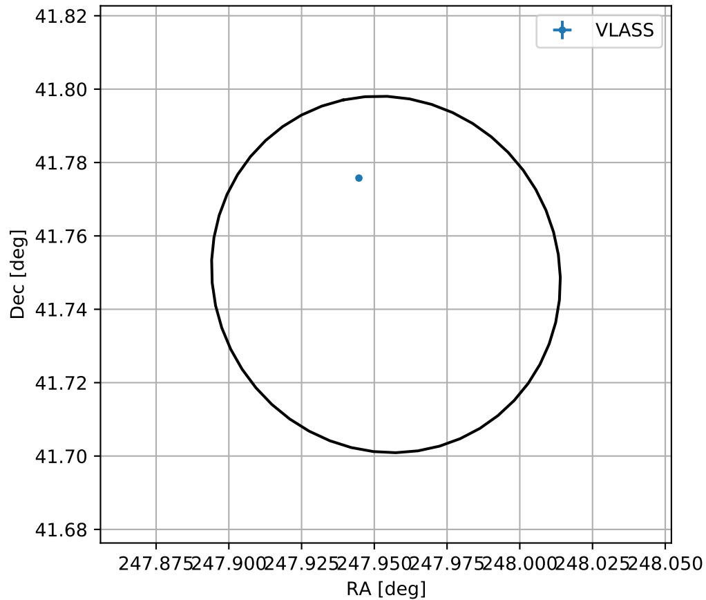
4FGL J1631.8+4144
