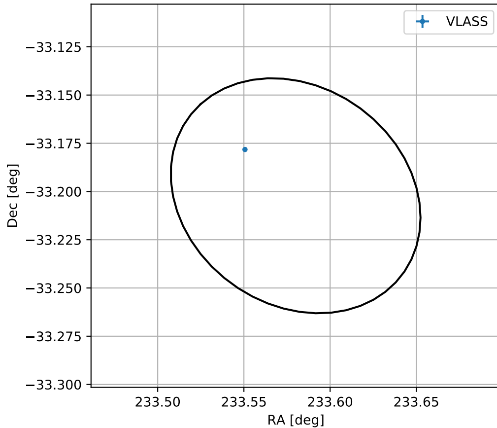
4FGL J1534.3-3312
