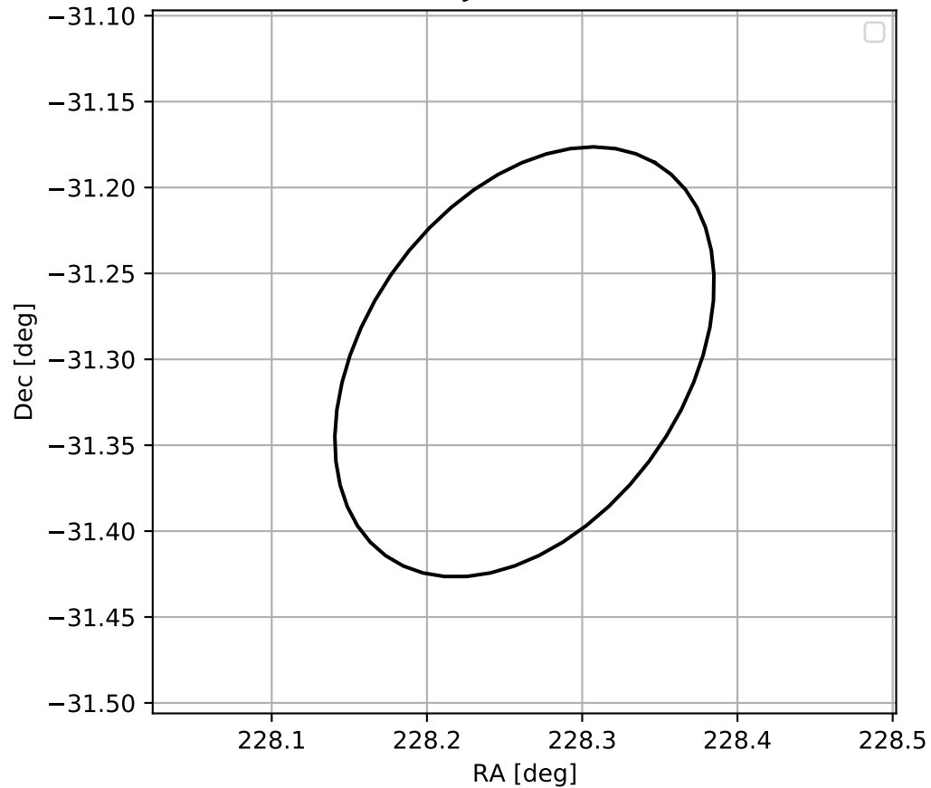
4FGL J1513.0-3118
