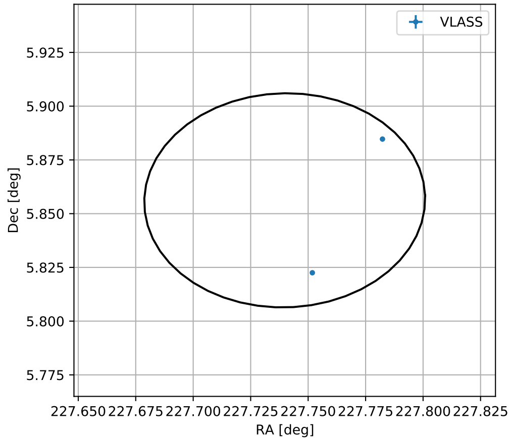
4FGL J1510.9+0551
