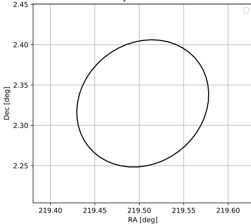
4FGL J1438.0+0219
