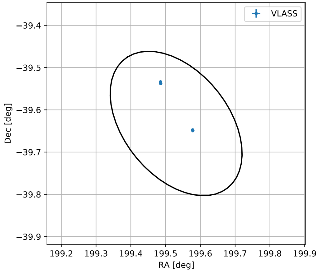
4FGL J1318.1-3937
