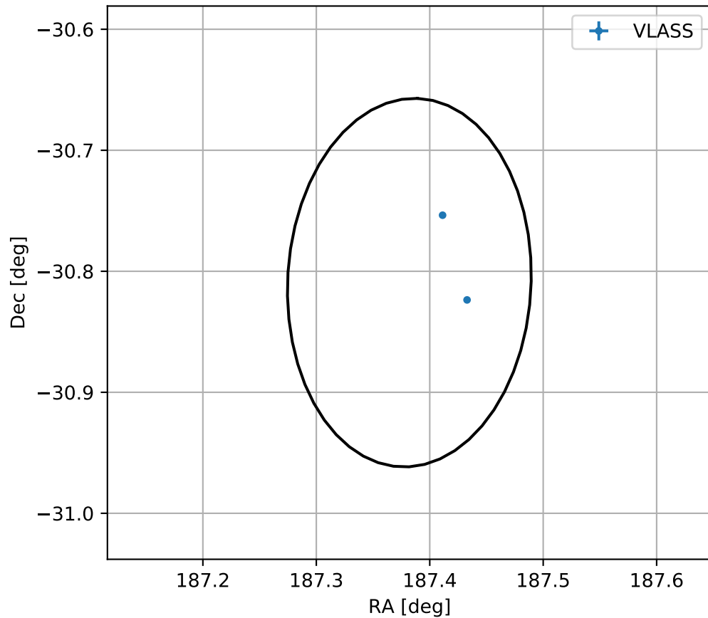
4FGL J1229.5-3048
