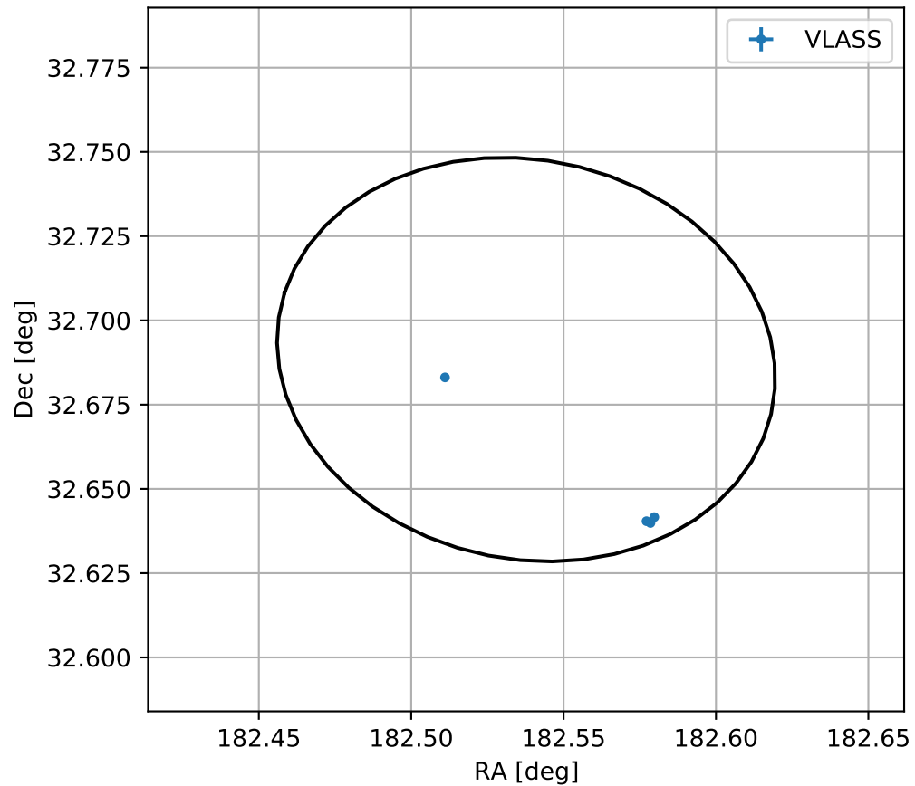
4FGL J1210.1+3241
