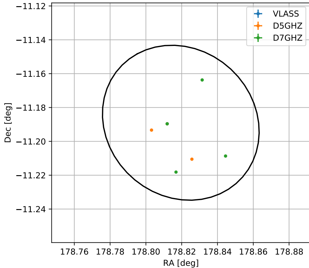
4FGL J1155.2-1111
