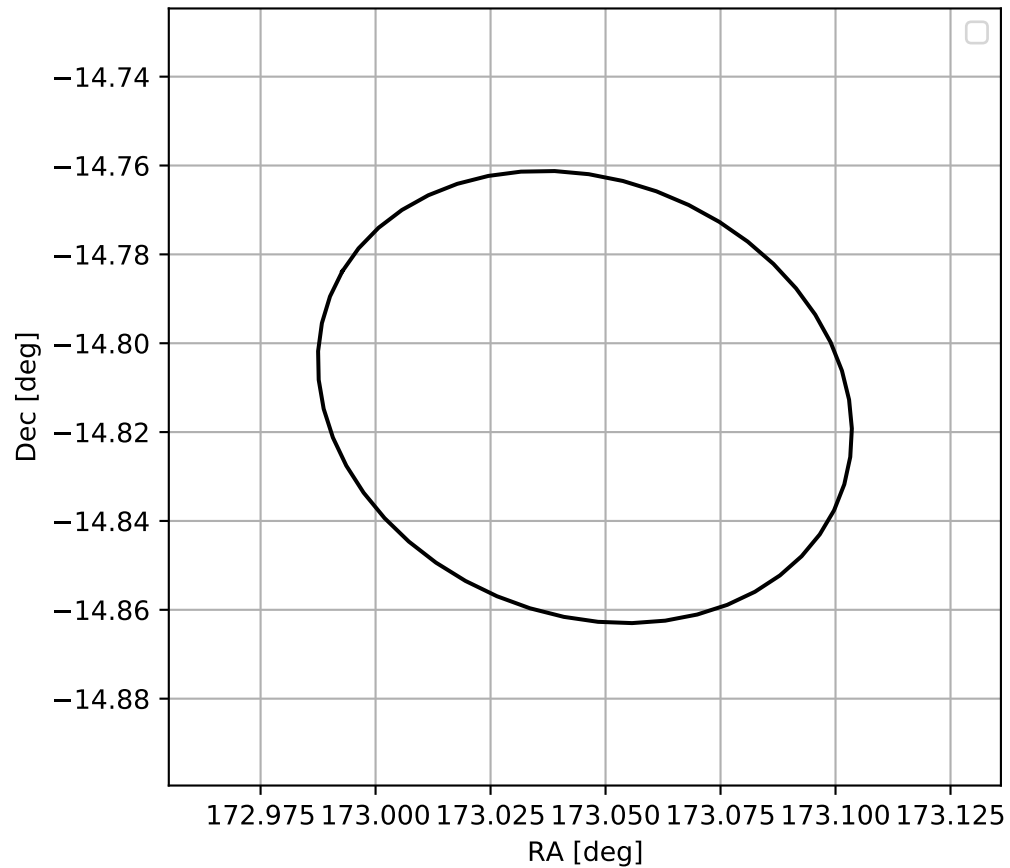
4FGL J1132.1-1448
