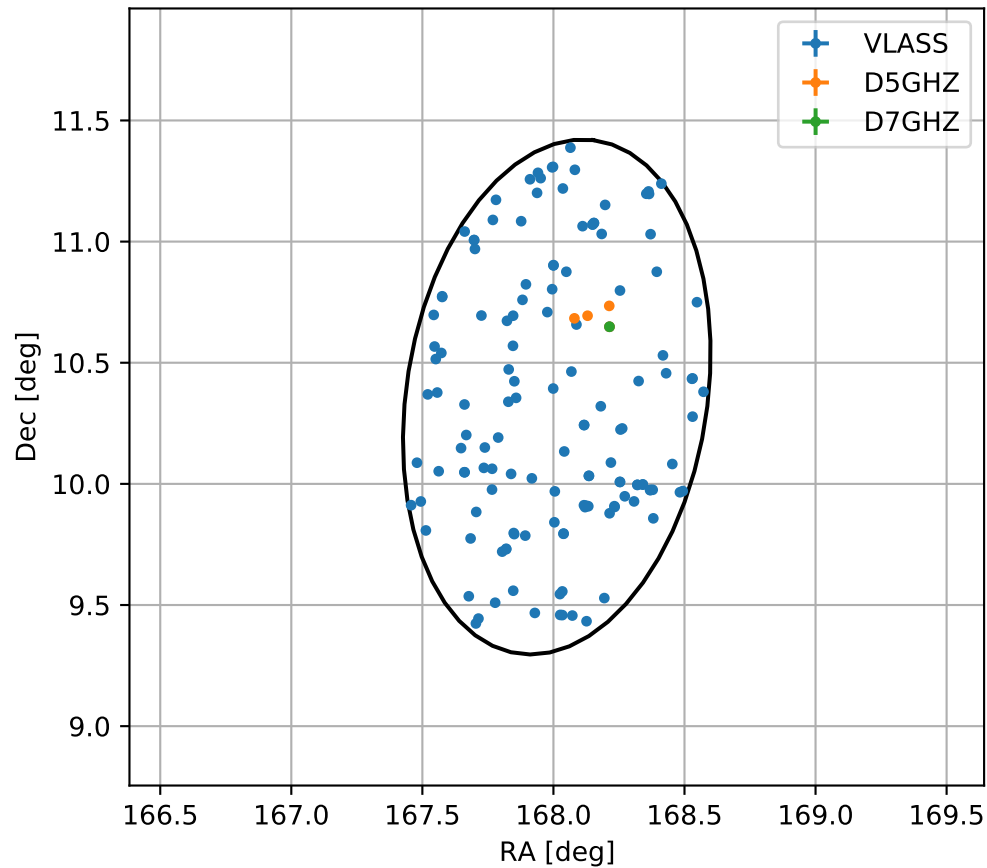
4FGL J1112.0+1021
