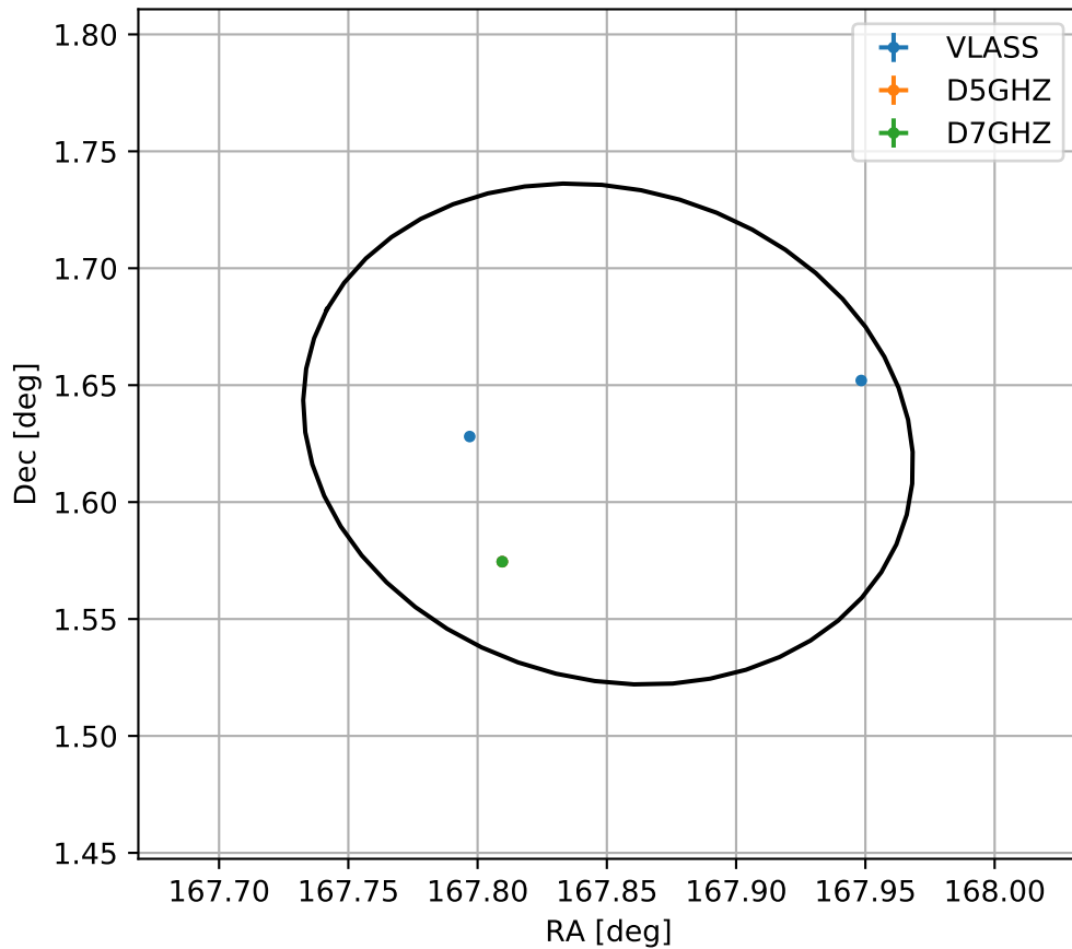
4FGL J1111.4+0137
