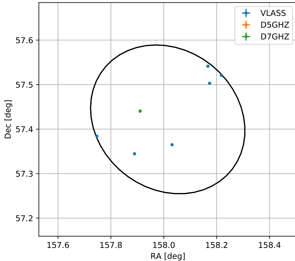
4FGL J1032.0+5725
