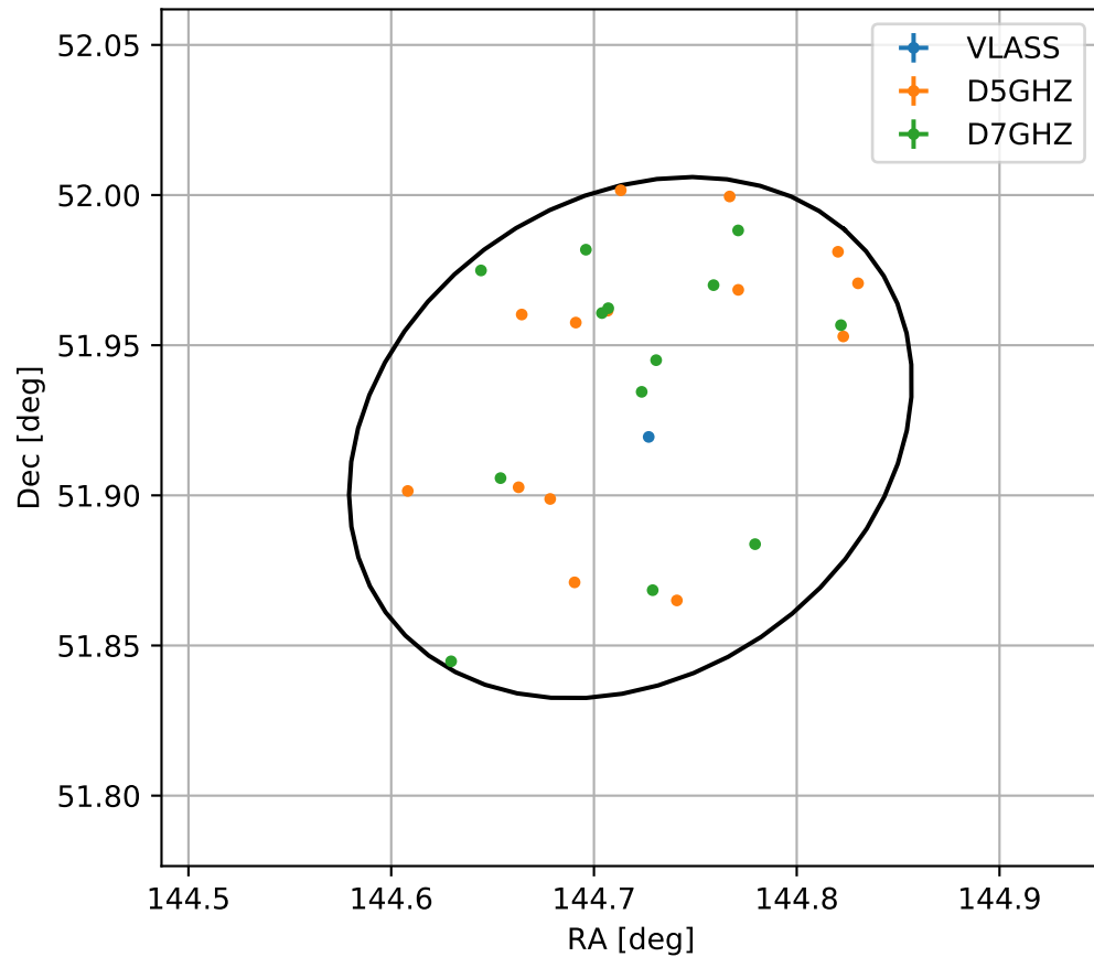
4FGL J0938.8+5155
