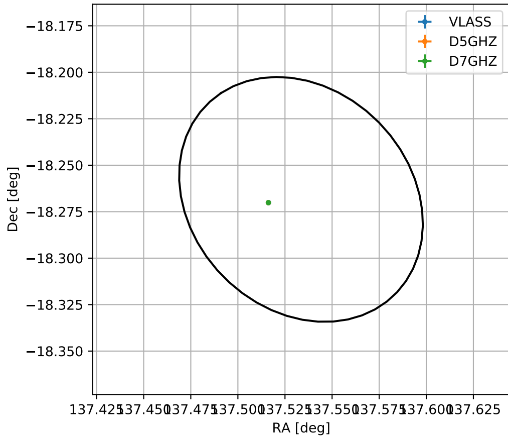
4FGL J0910.1-1816
