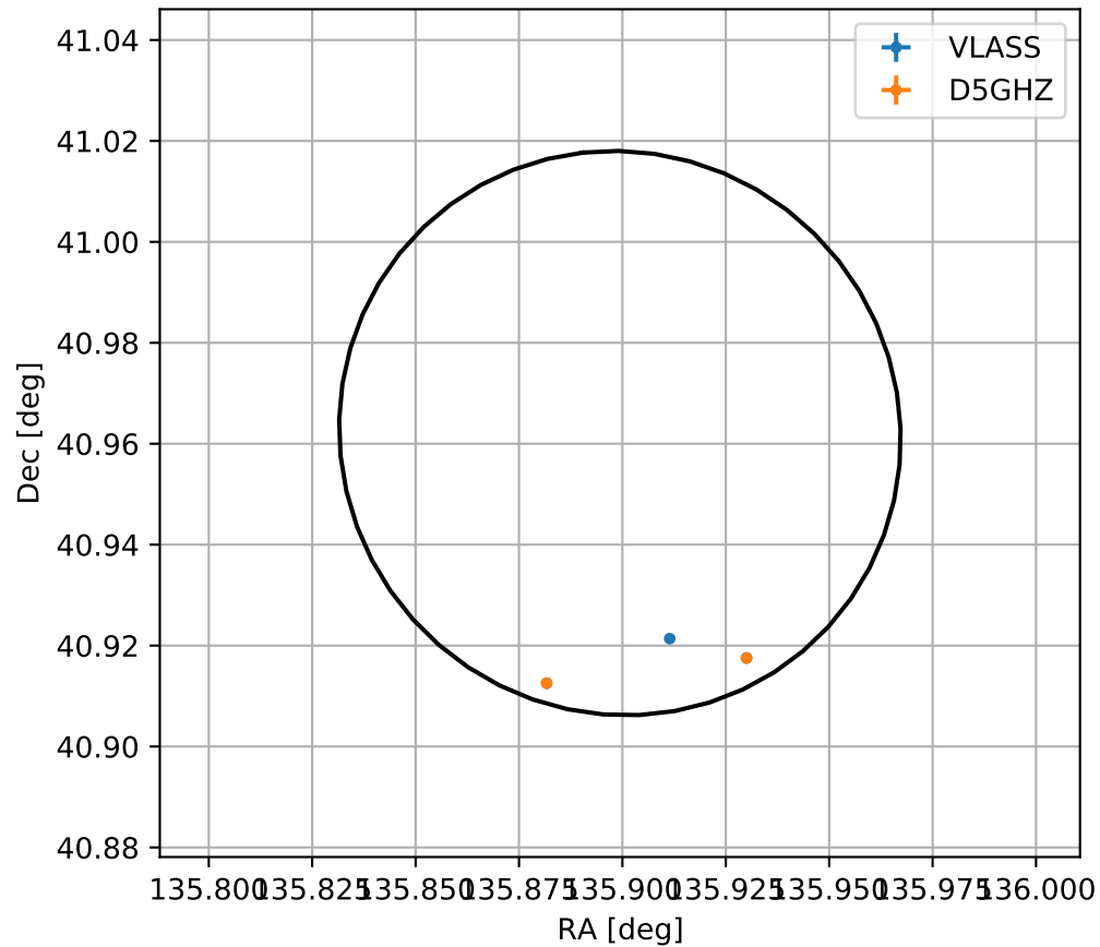
4FGL J0903.5+4057
