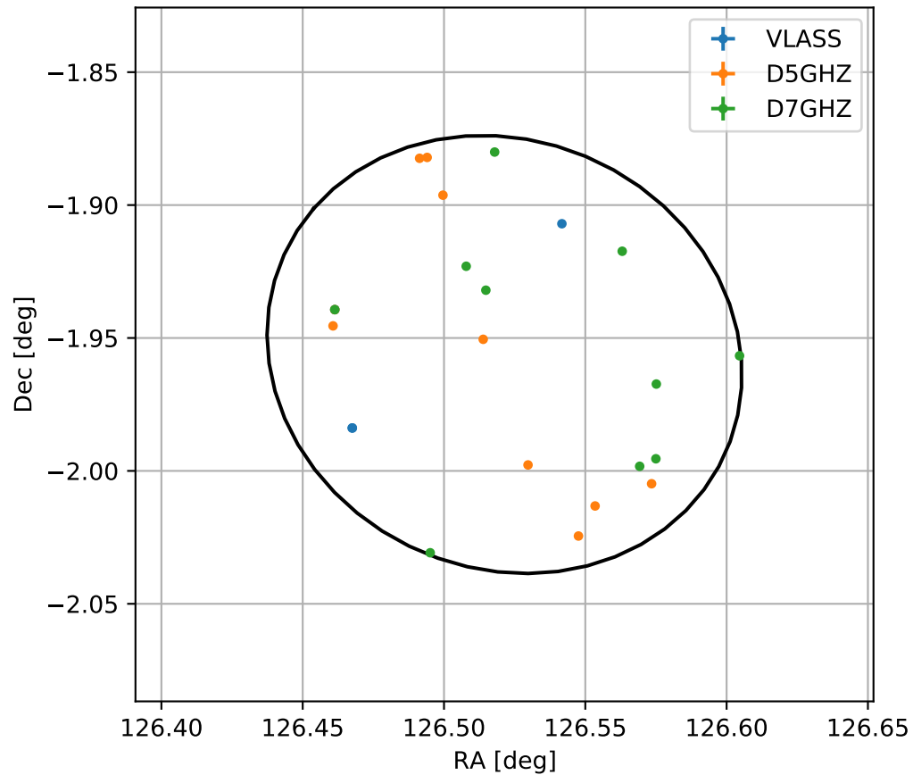
4FGL J0826.0-0157
