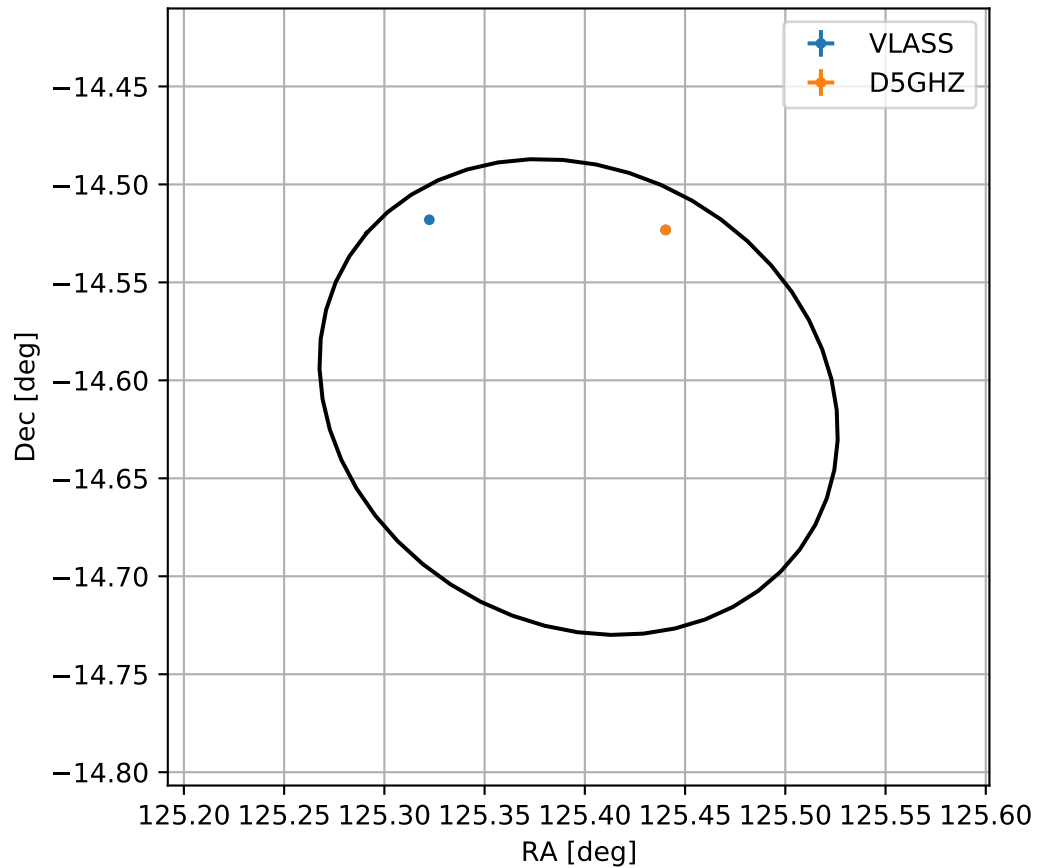
4FGL J0821.5-1436
