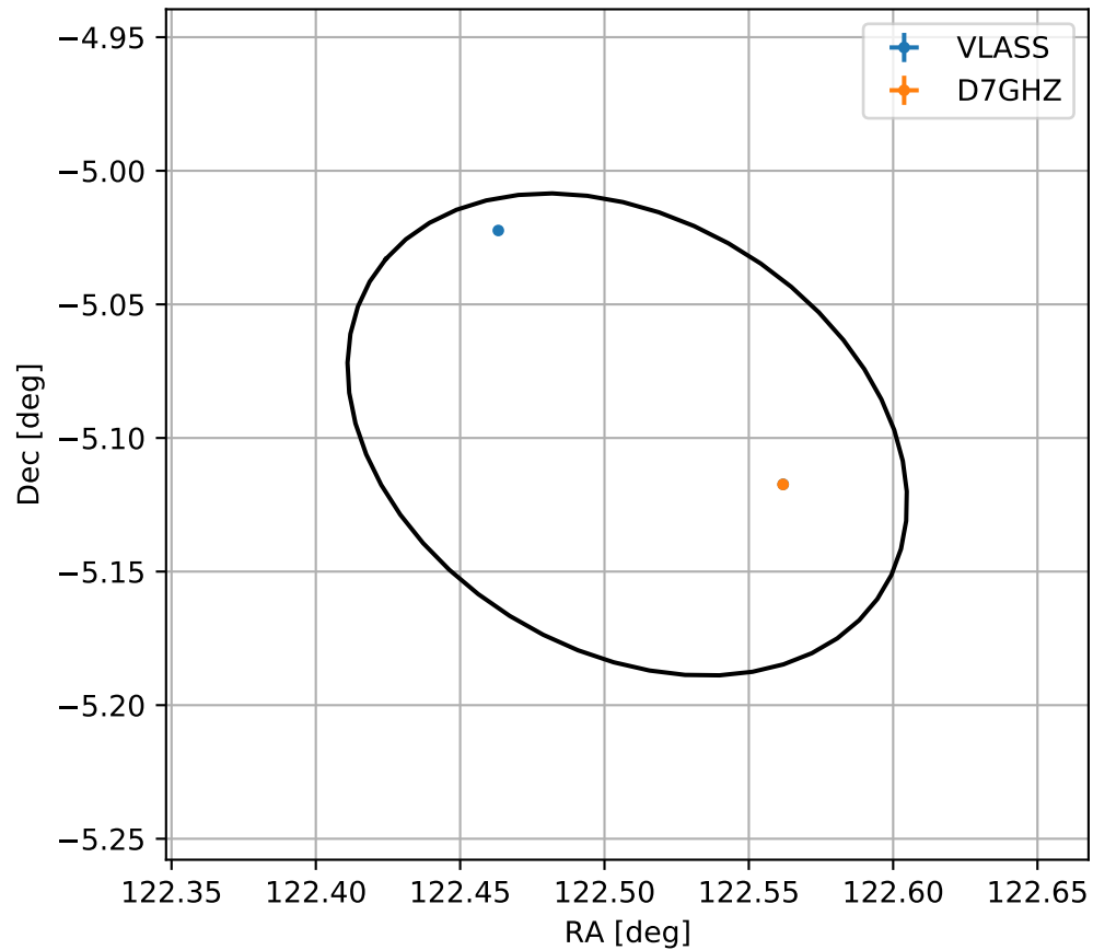
4FGL J0810.0-0505
