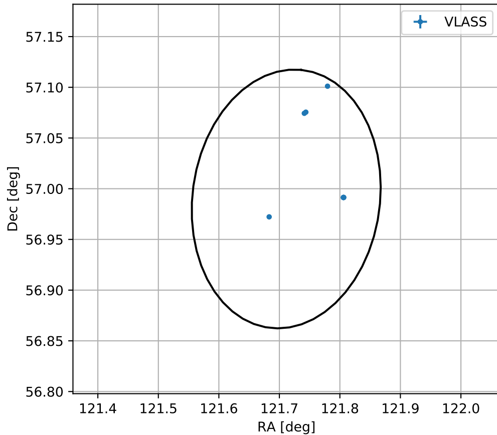
4FGL J0806.8+5659
