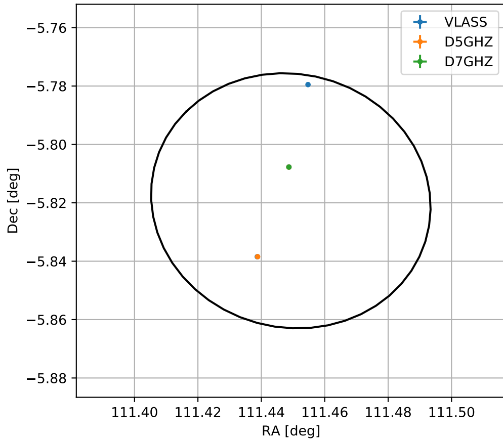
4FGL J0725.7-0549
