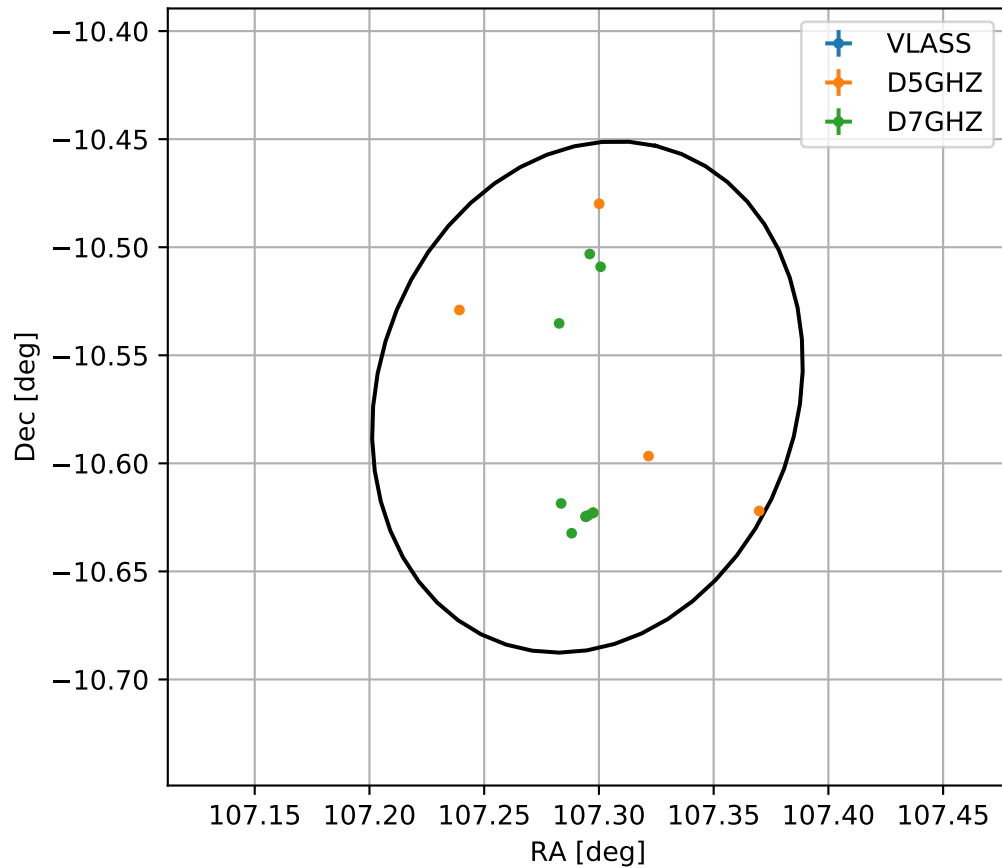
4FGL J0709.1-1034c
