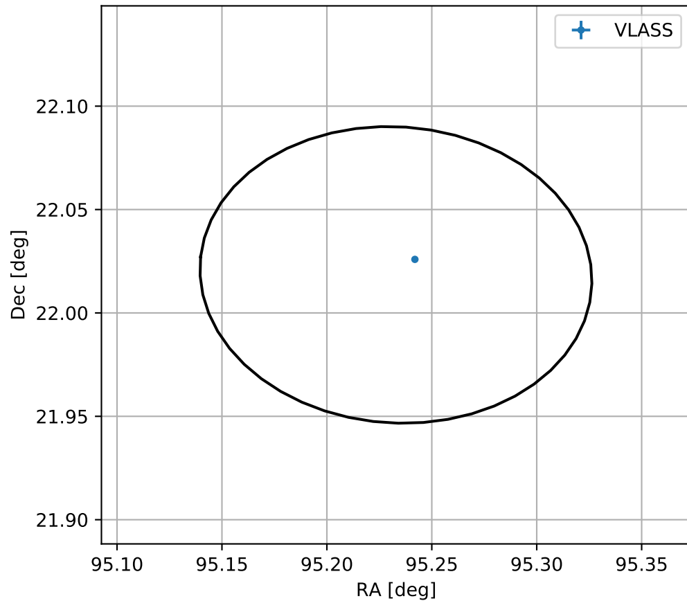
4FGL J0620.9+2201
