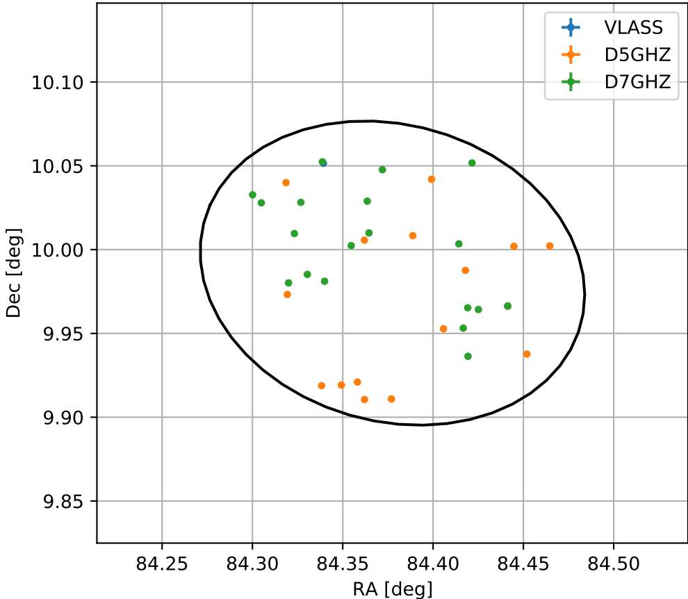
4FGL J0537.5+0959
