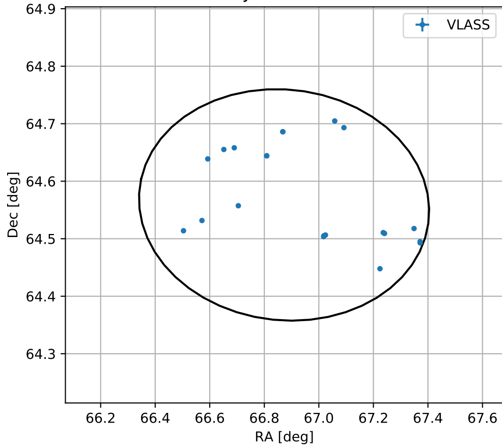
4FGL J0427.4+6433c
