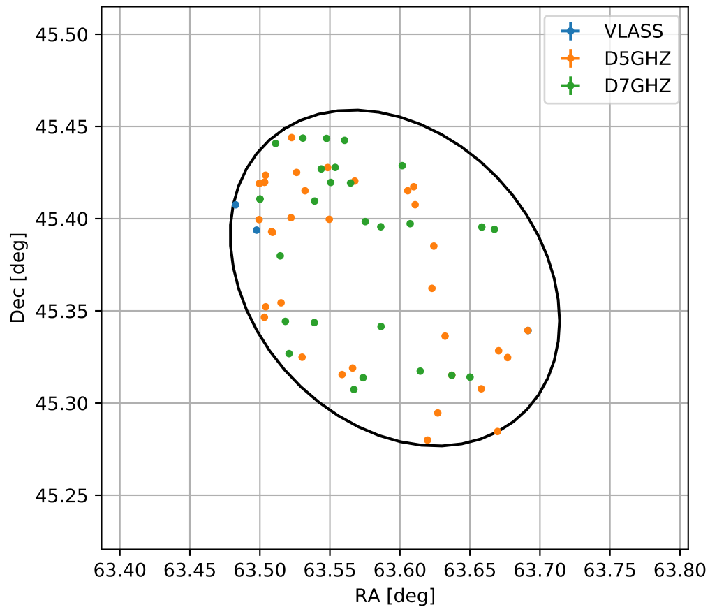
4FGL J0414.3+4522
