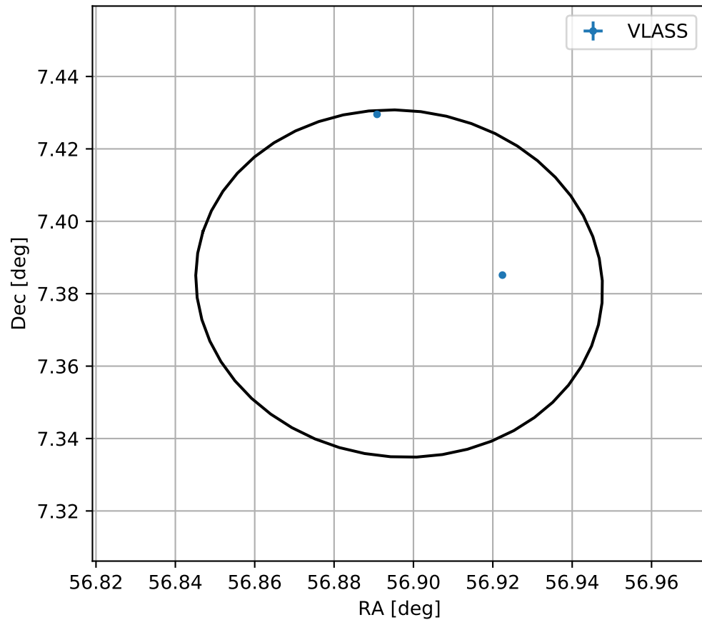
4FGL J0347.5+0722
