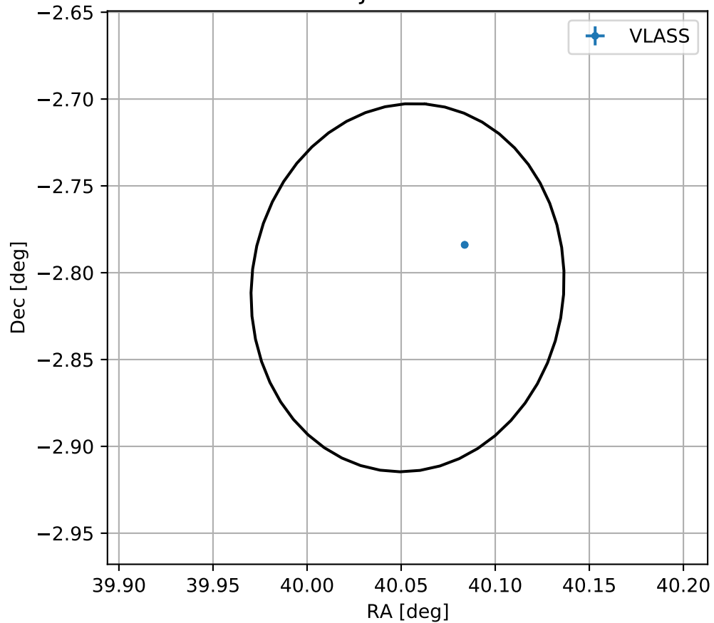
4FGL J0240.2-0248
