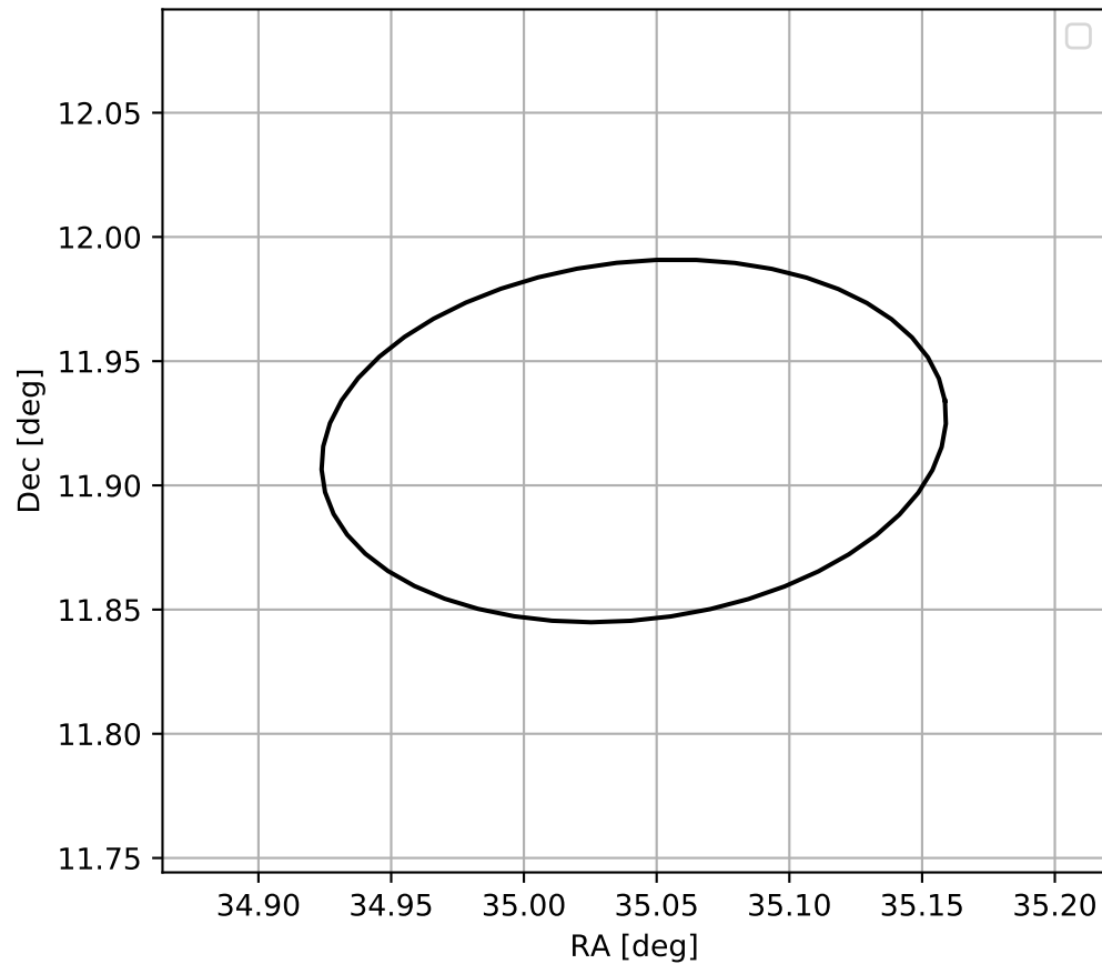
4FGL J0220.1+1155
