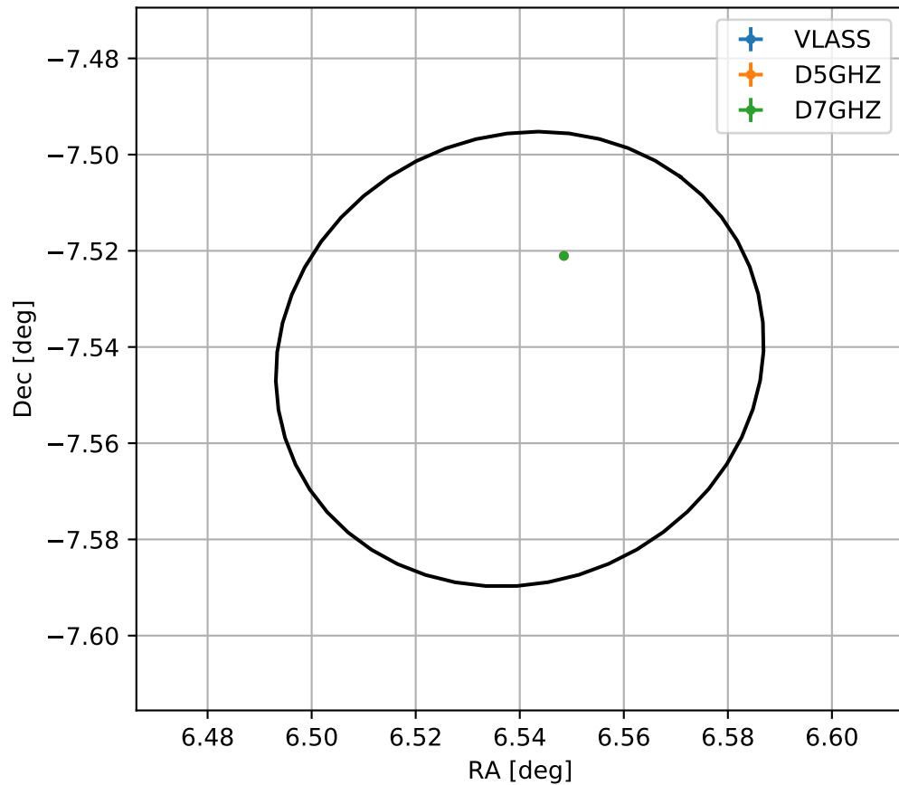
4FGL J0026.1-0732
