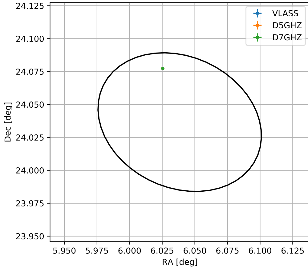
4FGL J0024.1+2402
