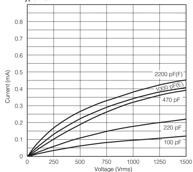
Type FC
